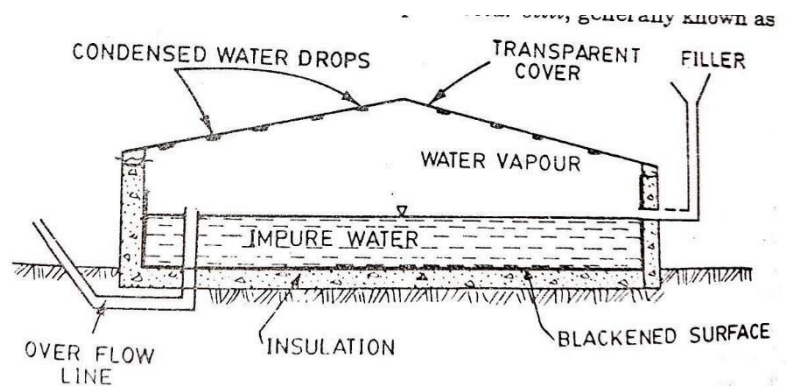
Fig. 5.8.1. Solar Water Still.
